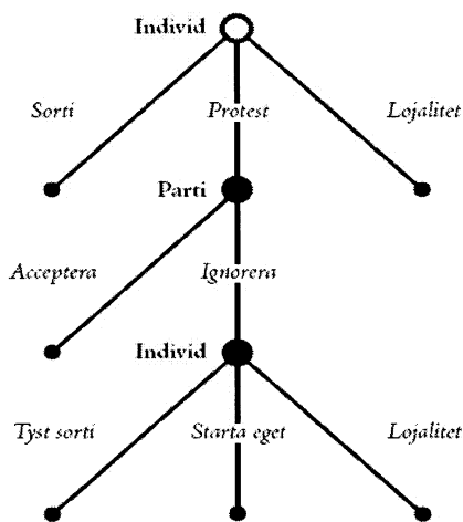
Figur 1. Den sekventiella modellen som spelträd.
